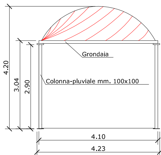
- PROSPETTO LATO 4 m
