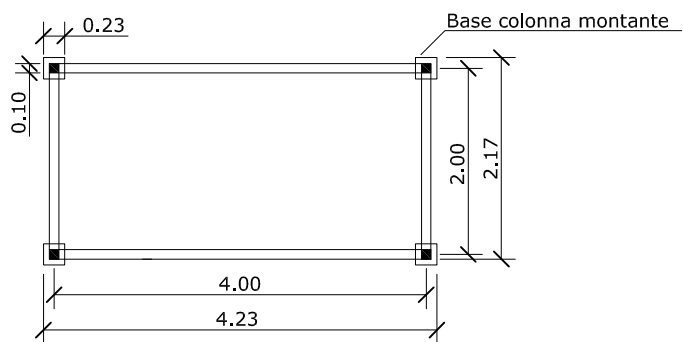
- PIANTA
